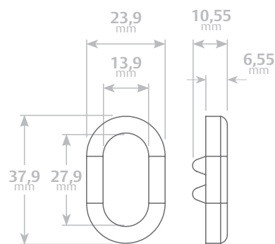
Espelho
