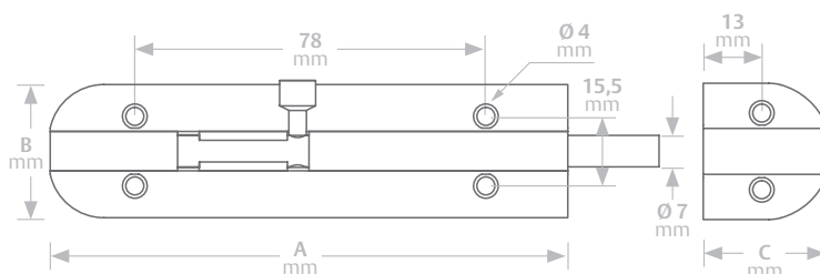
Ferrolho 545
