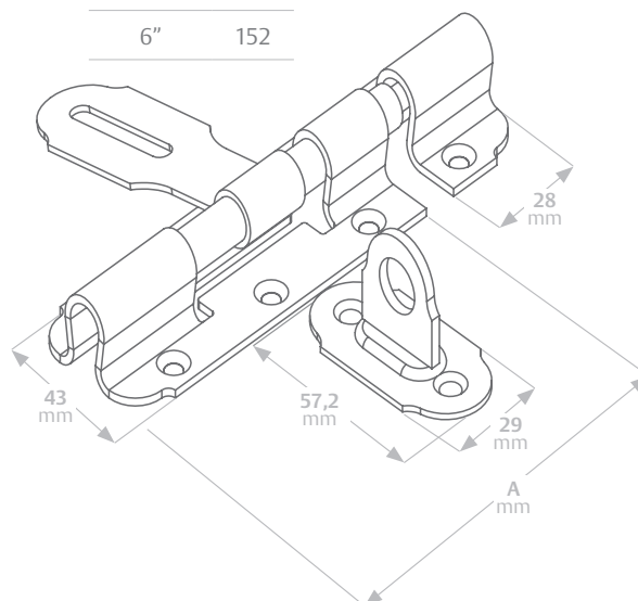
Ferrolho 545
