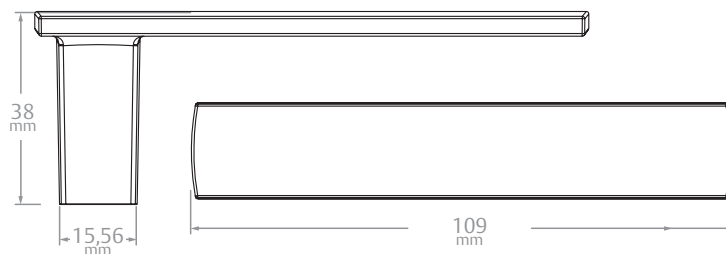
Maçaneta
